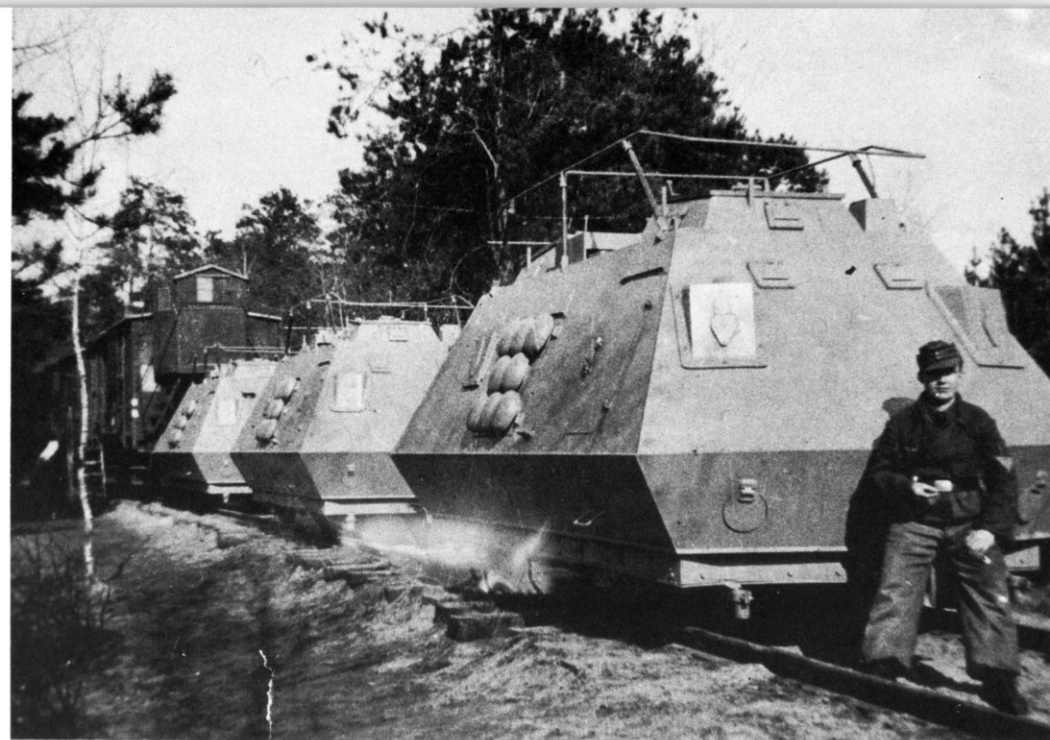
Drei der Wagen des leichten Spähzuges Nr. 303. Der gesamte Zug bestand aus zehn dieser Fahrzeuge, die meist als Einzelfahrer, jedoch paarweise (zu gegenseitiger Hilfe) eingesetzt wurden. (SA)
