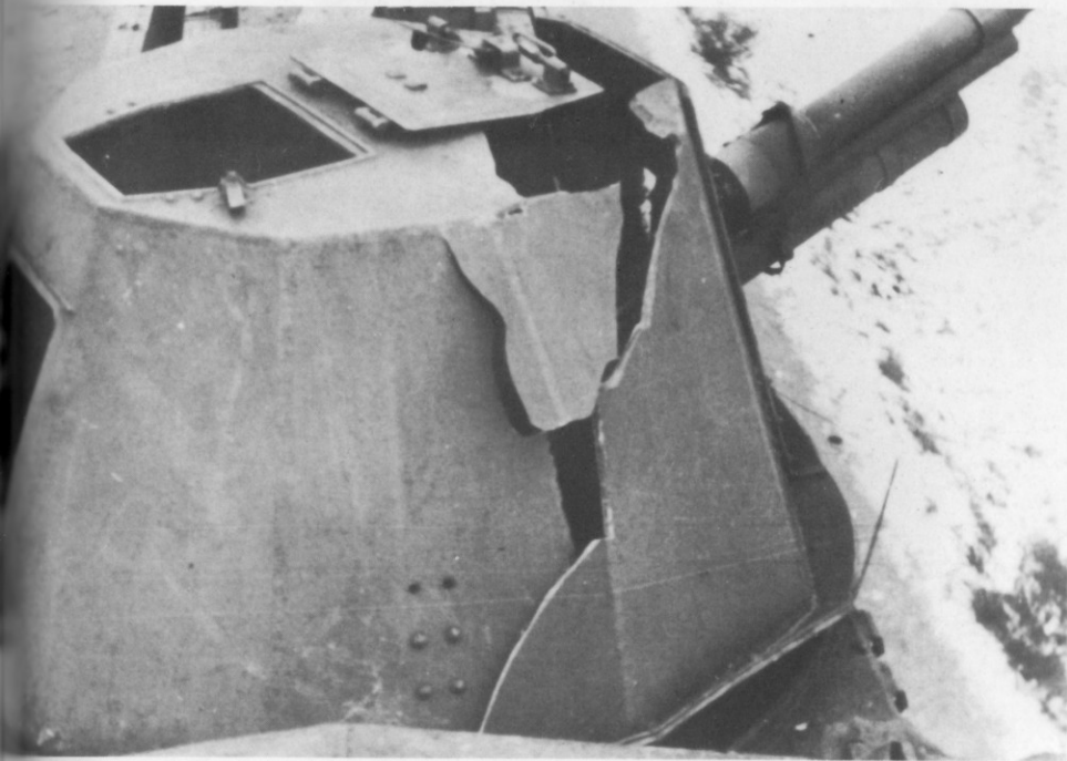
Oben: Ein Rohrkrepiierer zerriß beim Panzerzug Nr. 67 nicht nur den Lauf der 7,62-cm-F.K. 295/1(r), sondern sprengte auch den Panzerturm. Unten: Nachdem der Panzerzug Nr. 1 vorher schon im Kampfeinsatz beschädigt worden war, traf ihn am 10. 12. 1942 in Wjasma auch noch eine Bombe. Daraufhin erfolgte sein Neubau im RAW Königsberg. (SA)
